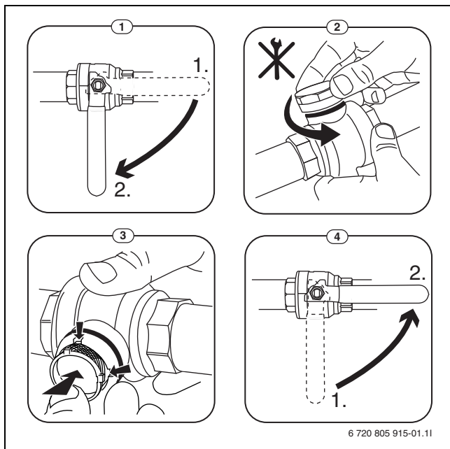
Afb. 7 Filterreiniging
