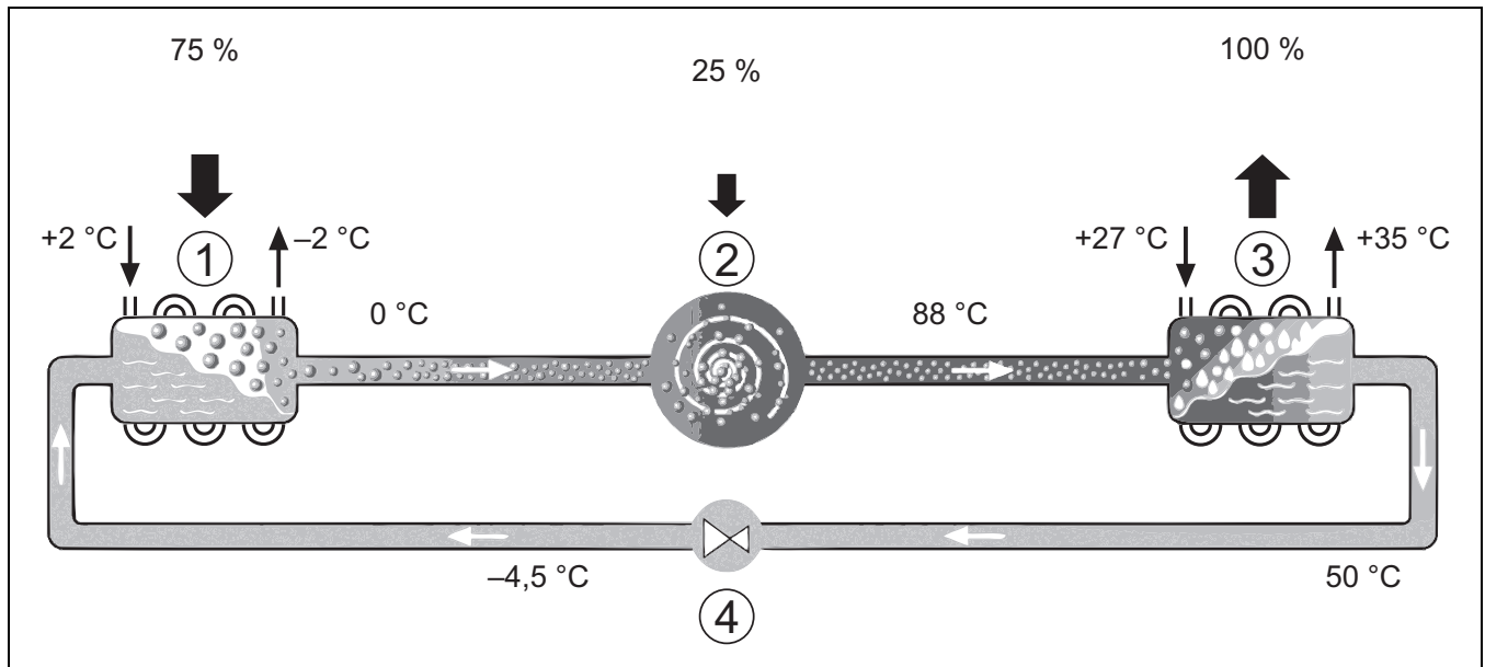
Afb. 1 Werkingsprincipe van het koudemiddelcircuit in de warmtepomp
